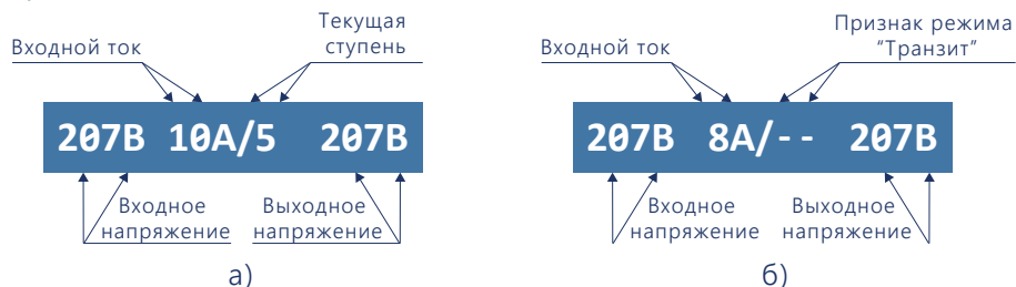
Рисунок 5.2 - Примеры изображений на индикаторе стабилизатора («начальный экран») а) в режиме «Стабилизация»; б) в режиме «Транзит»
